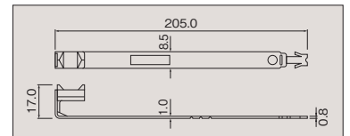
(ポリプロピレン) 結束径: 95mm φ
