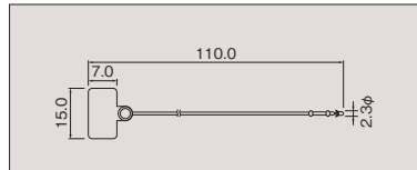
(ポリプロピレン) 結束径: 30mm φ
