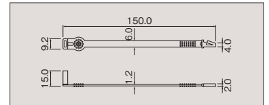
(ポリプロピレン) 結束径: 45mm φ
