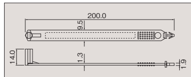
(ポリプロピレン) 結束径: 60mm φ
