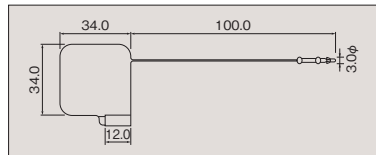
(ポリプロピレン) 結束径: 35mm φ
